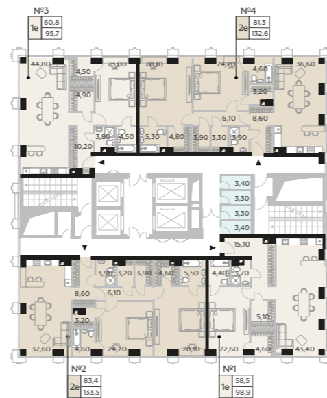
Корпус 2 (52 этажа)
